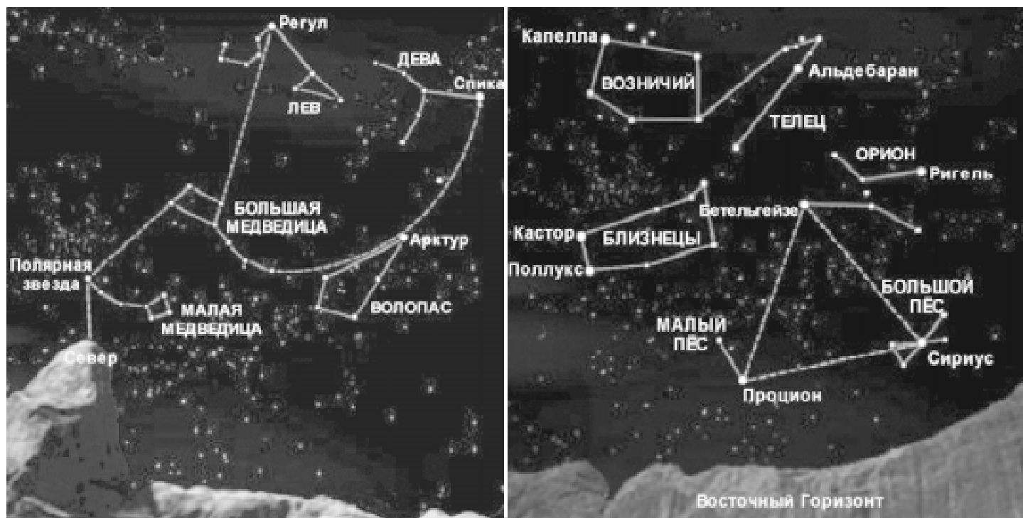
Наиболее яркие звезды, которые имеют свои собственные имена
